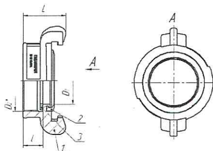
1 – корпус; 2 – кольцо уплотнительное; 3 – прокладка
