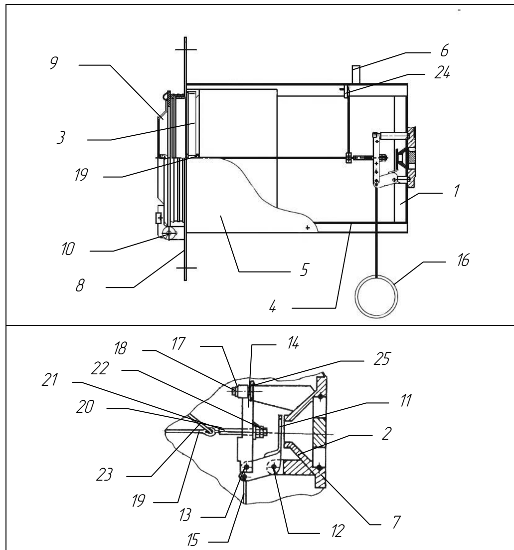
Рисунок 1 - Устройство генератора ГПС
