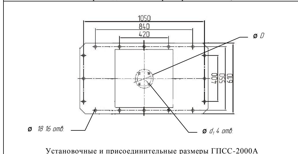
Установочные и присоединительные размеры ГПСС-600, ГПСС-2000
