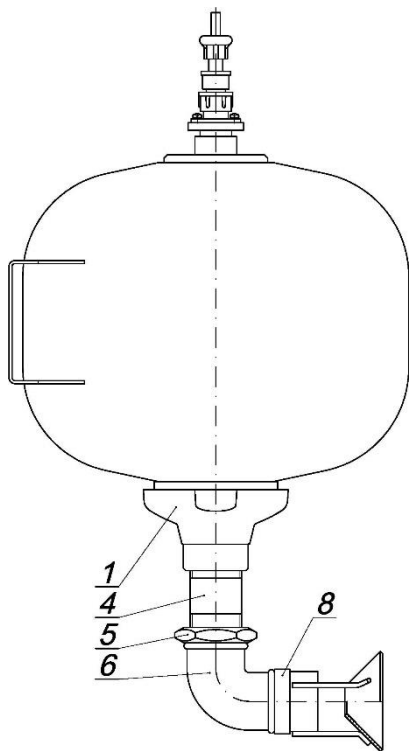
Рисунок 3 – Пример монтажной схемы направляющего трубопровода модуля Буран-15КДН или Буран-15КДТ
