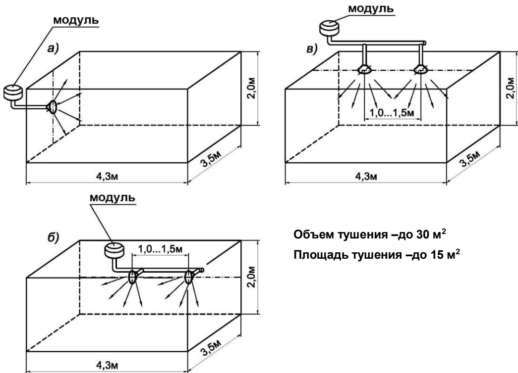
Рисунок 2 - Масштабное изображение области, в которой достигаются условия тушения модулями Буран-15КДН и Буран-15КДТ по очагам класса А и В
