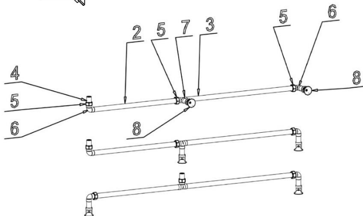
направляющего трубопровода модулей Буран-15КДН или Буран-15КДТ
