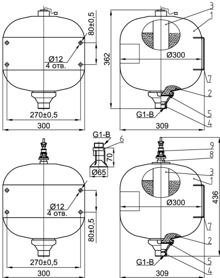
Рисунок 1 - Устройство модуля
